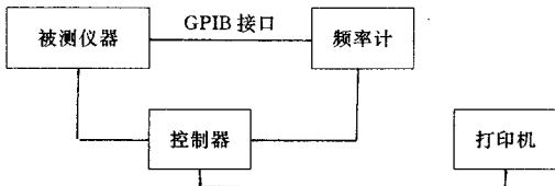
图 4 多频仪器测试信号频率测试系统示意图
